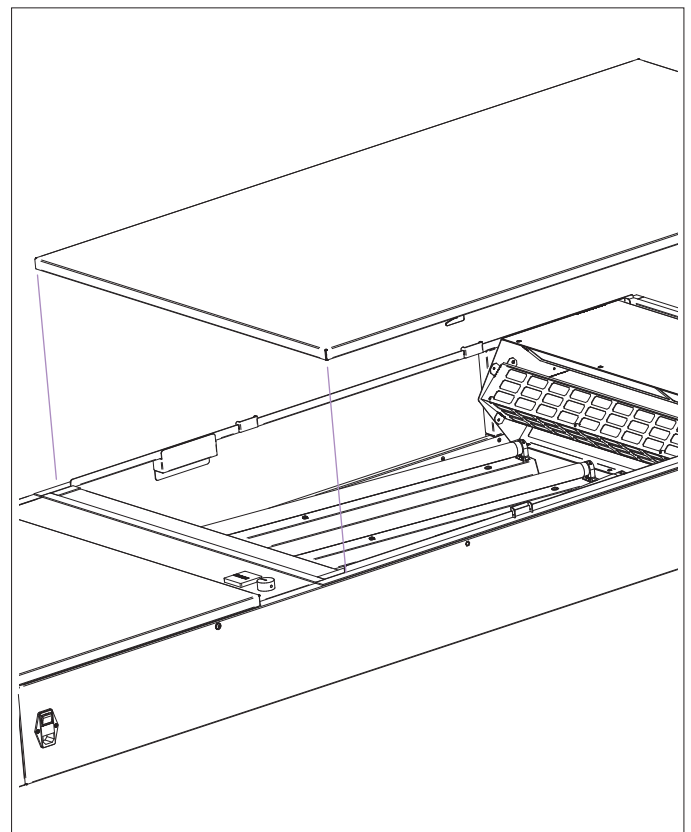
Entfernen Sie die UV-Reaktortür, nachdem Sie die Sicherungsschraube entfernt haben
