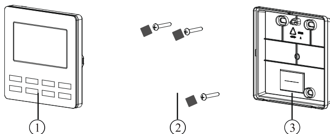
Abb. 22: Bauteile der Kabel-Fernbedienung
