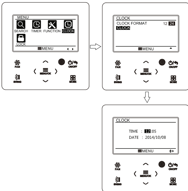
Abb. 19: Uhrzeit einstellen
